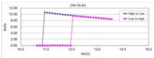
CHB200W12-72SXX-CMFD Iin Vs Vin
